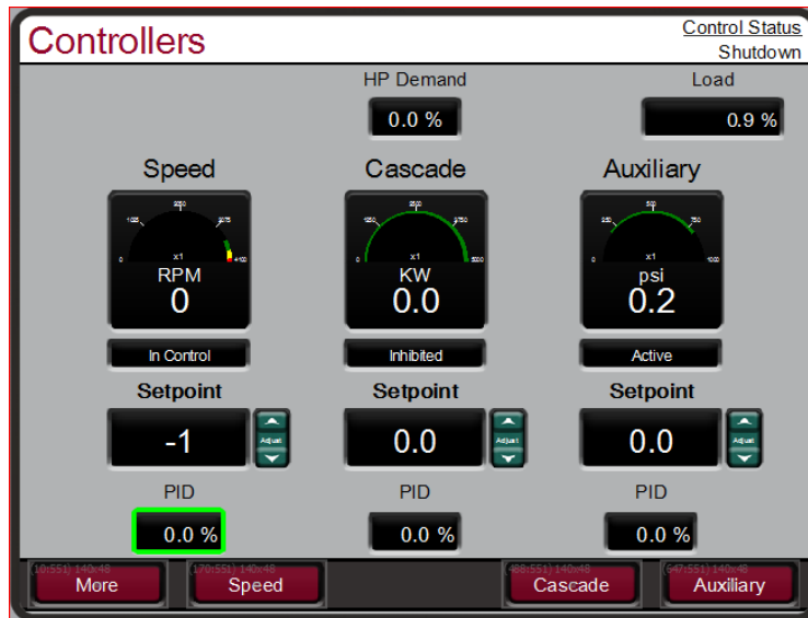
图 5-13.控制器屏幕
