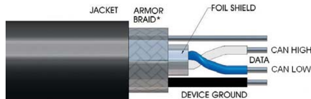
Belden YR58684, 散装电缆（伍德沃德件号 2008-1512）
