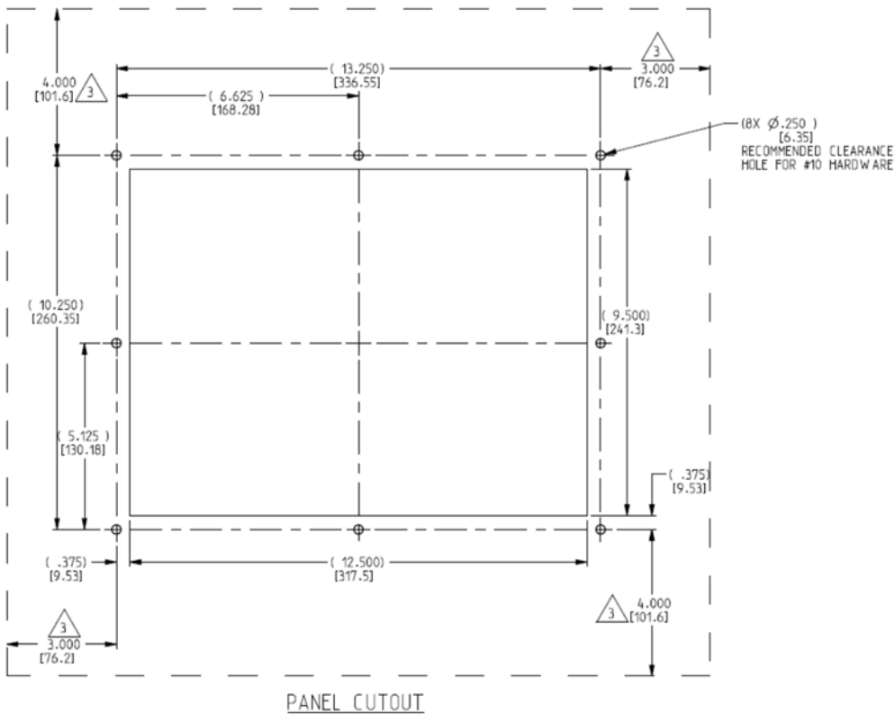
图 2-2.505D 外形图
