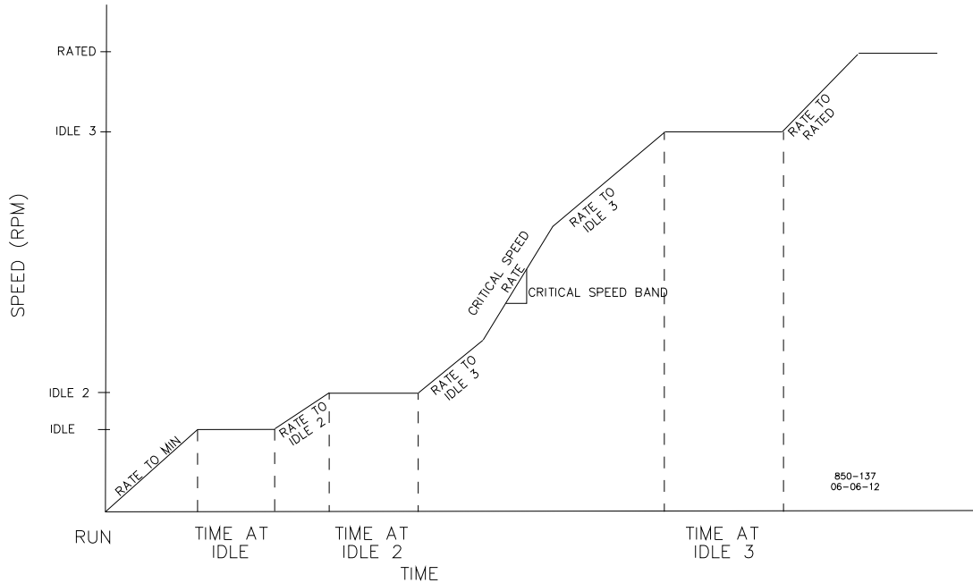
图 3-6.顺序自动启动
