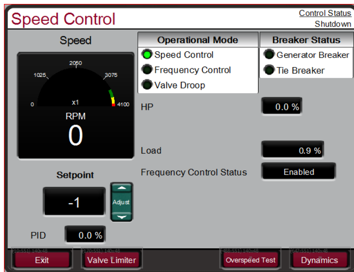
图 5-11.转速控制屏幕
