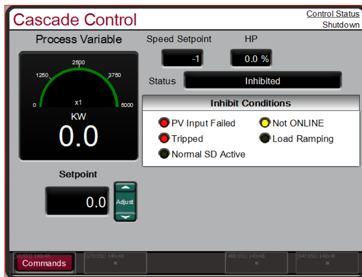
图 5-14.串级控制屏幕
