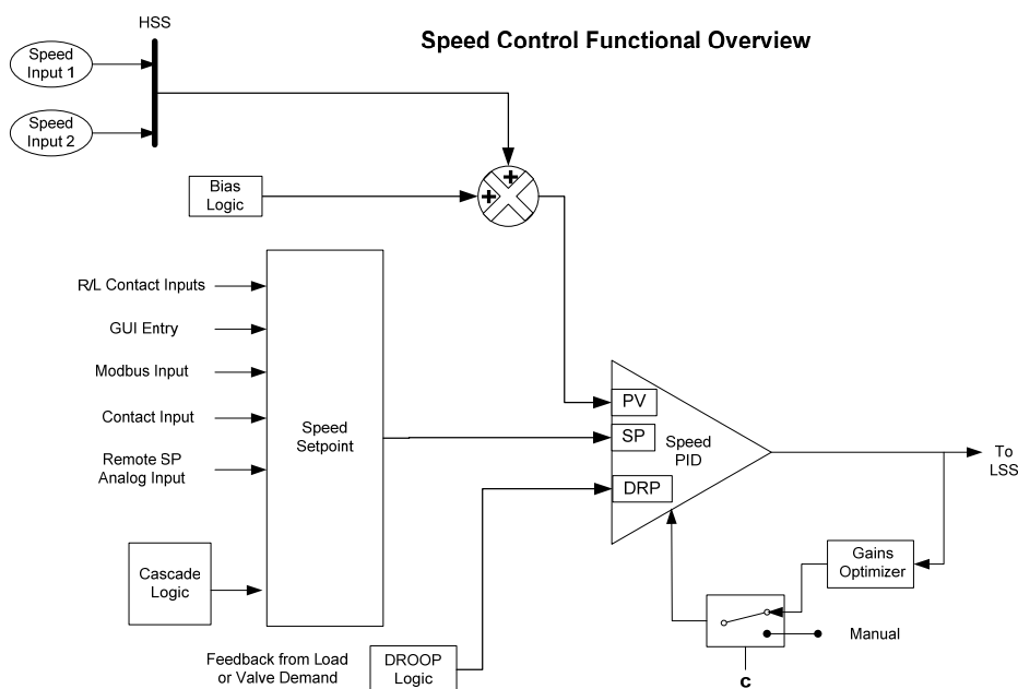
图 3-7.转速控制功能框图
