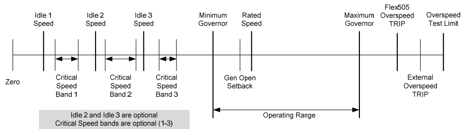
图 3-10. 转速关系
