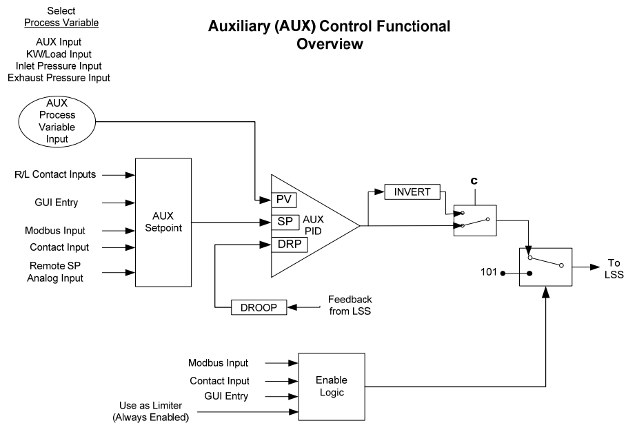
图 3-14. 辅助控制概述
