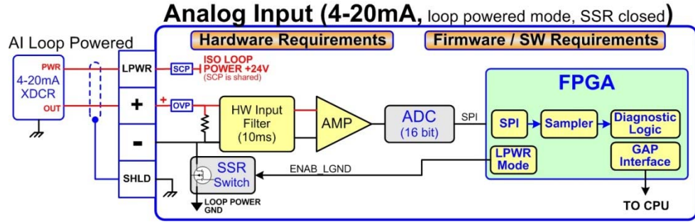
图 2-13. 模拟输入——环路供电框图
