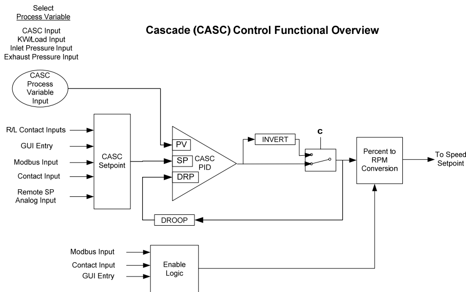
图 3-13.串级功能图
