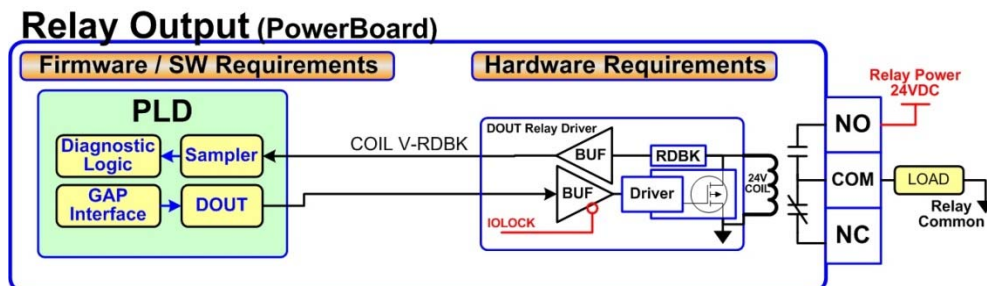
图 2-17.继电器输出框图
