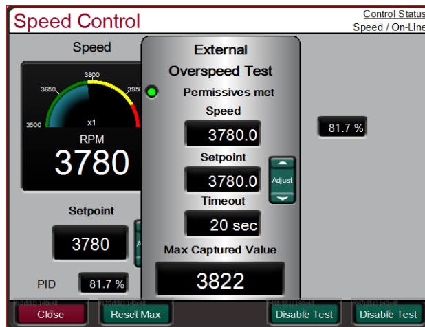
图 5-24.外部超速测试
