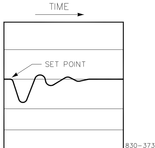
图 5-28.对负荷变化的典型响应
