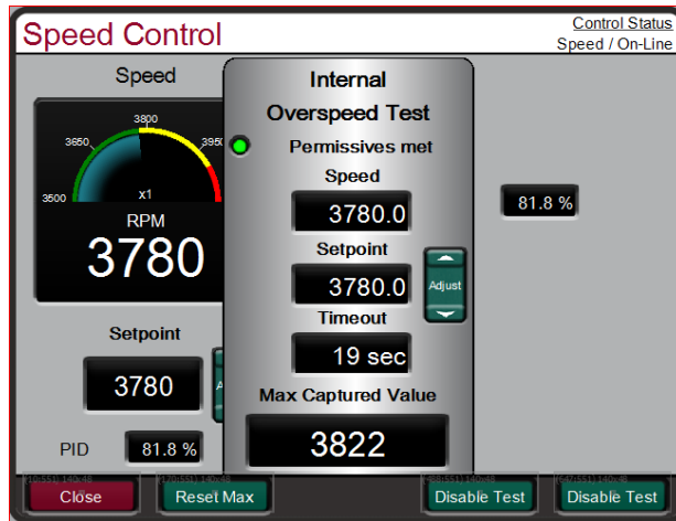
图 5-23.内部 (505) 超速测试
