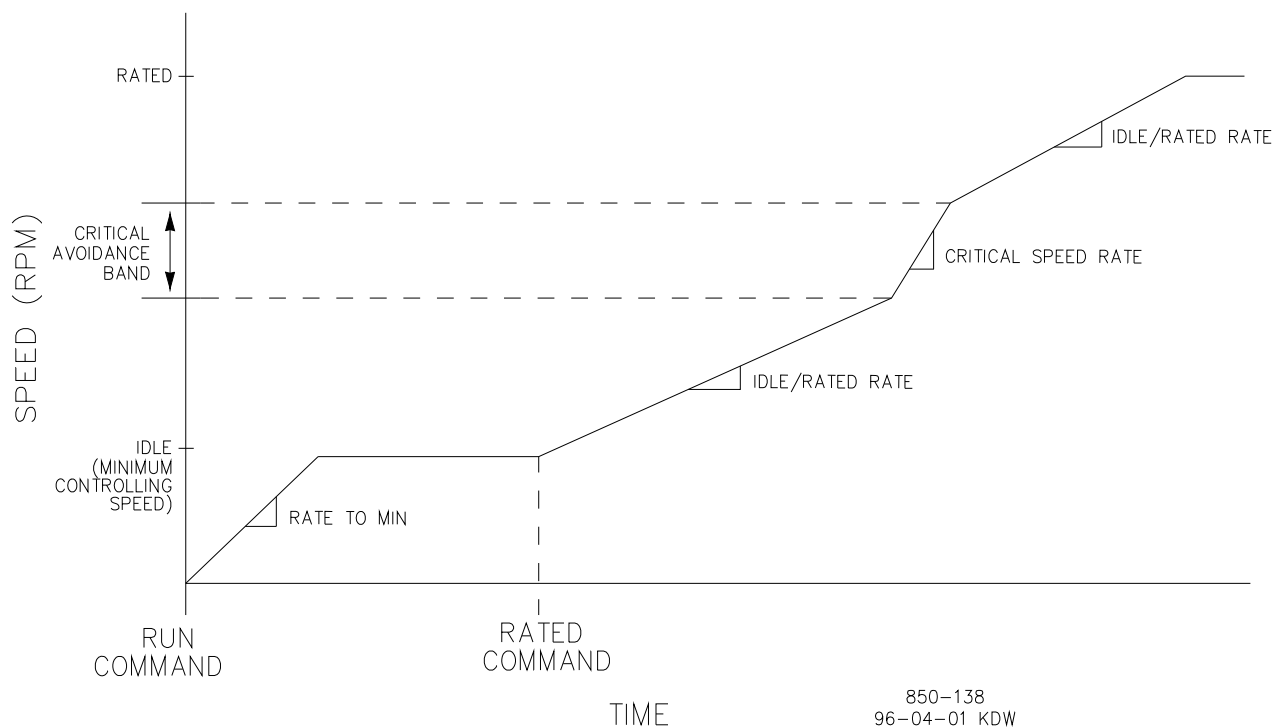
图 3-5.暖机/额定转速启动
