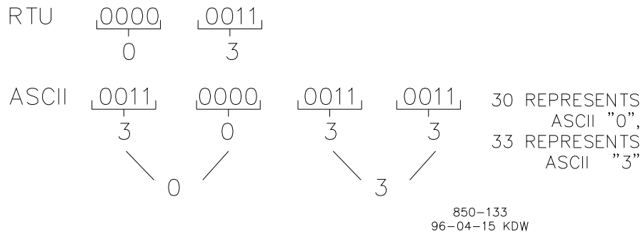
图 6-1.ASCII/RTU 模式下对 3 的表示
