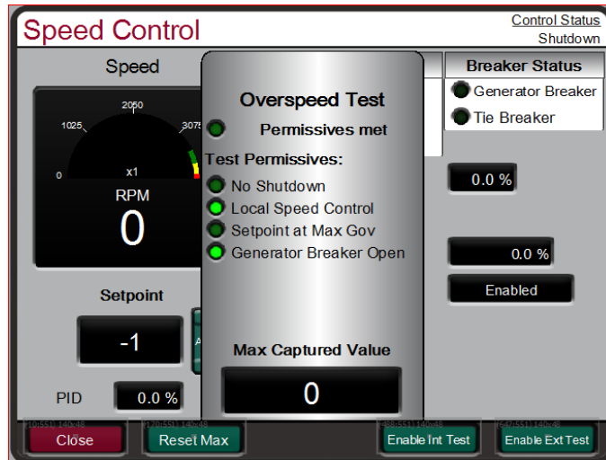
图 5-22.超速测试允许条件
