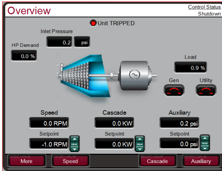
图 5-10.概览屏幕
