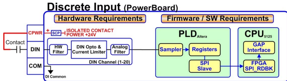
图 2-16.离散输入框图
