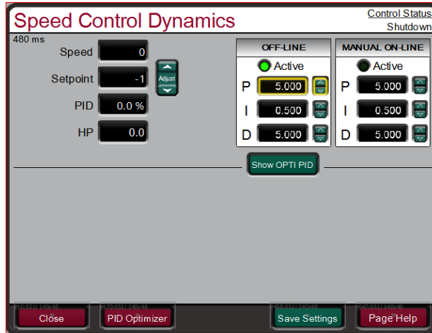
图 5-27.转速动态调整屏幕
