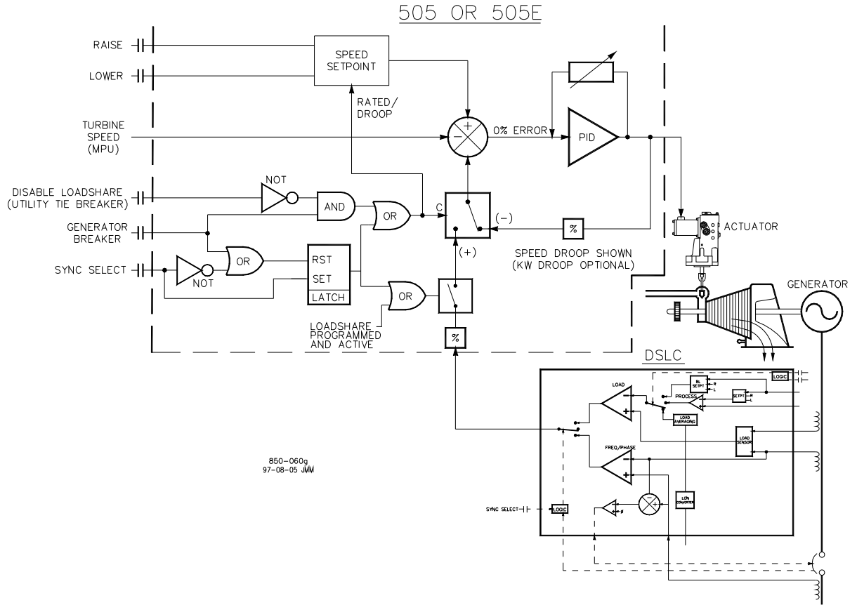
图 3-11. 负荷分配逻辑
