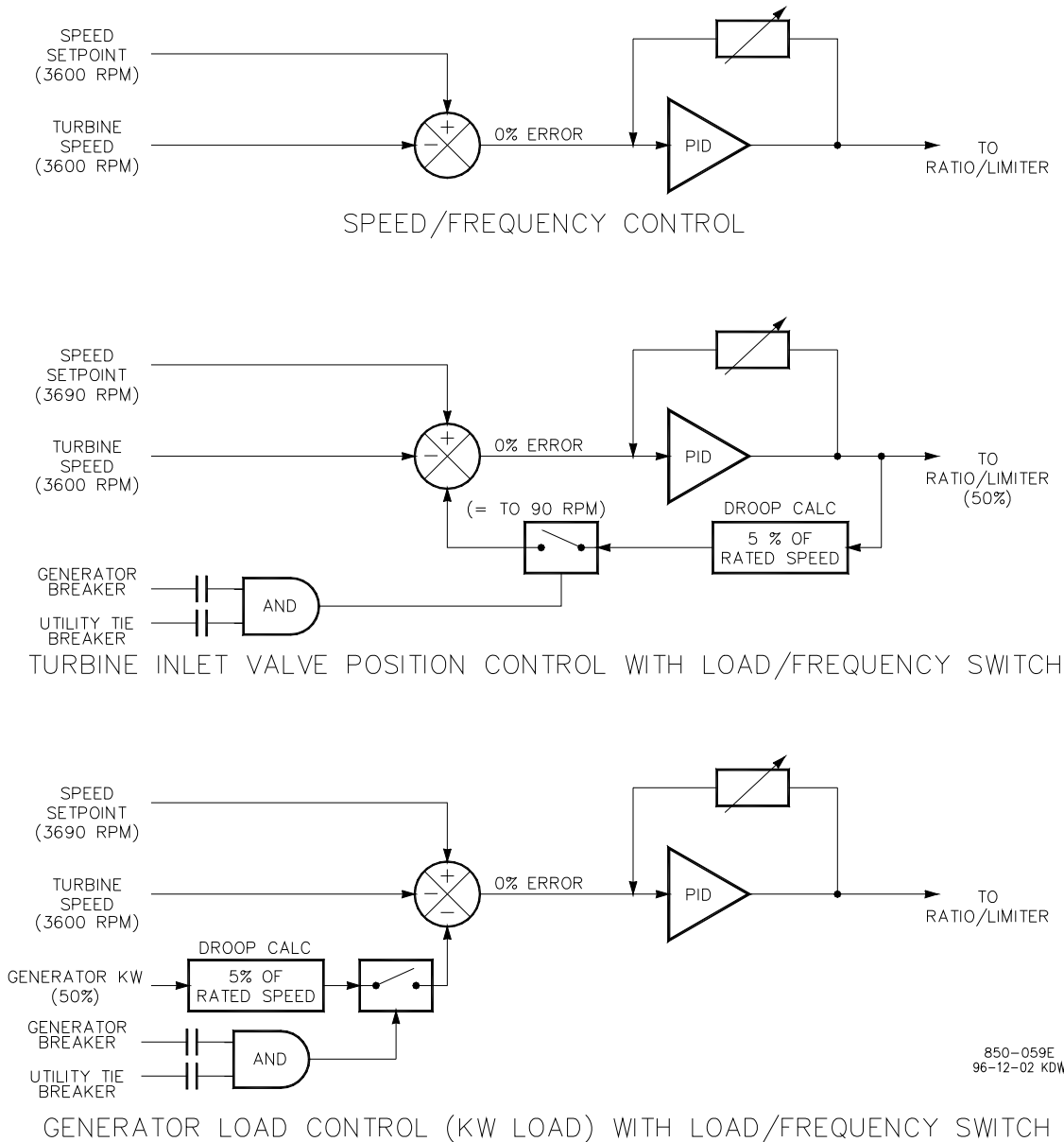
图 3-8.转速 PID 控制模式
