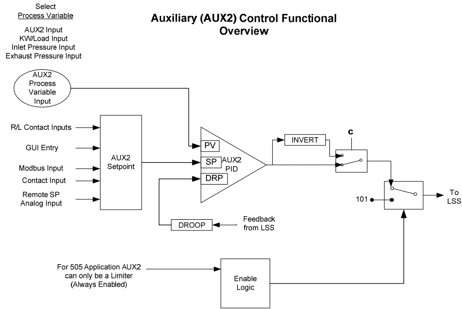
图 3-15.辅助 2 控制概述
