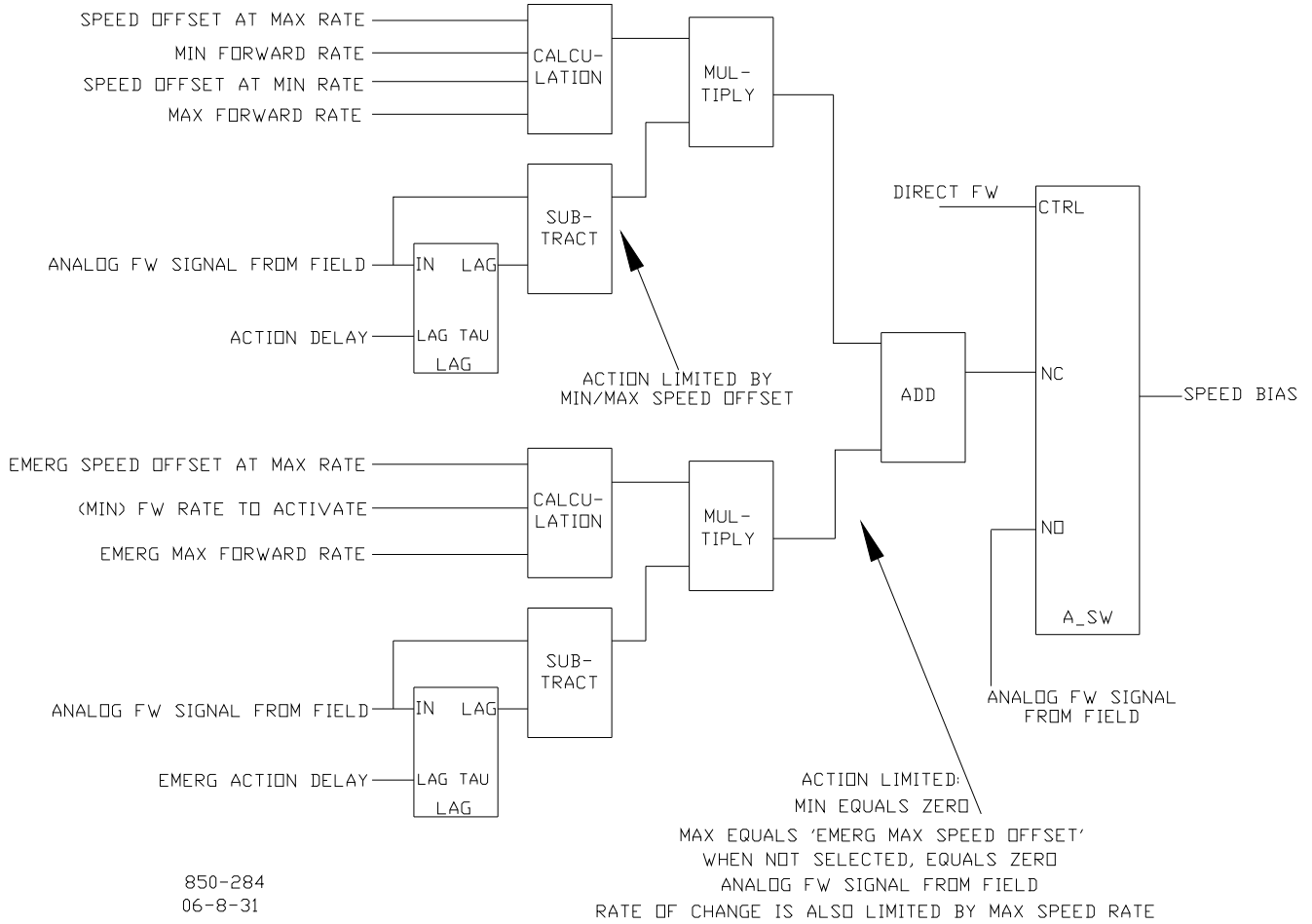
图 3-12.典型的防喘振阀和转速前馈逻辑趋势
