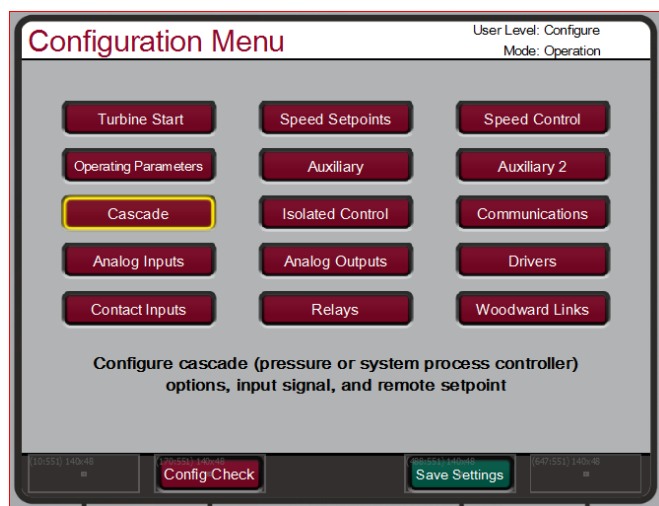
图 5-8.配置菜单——操作模式（仅查看）
